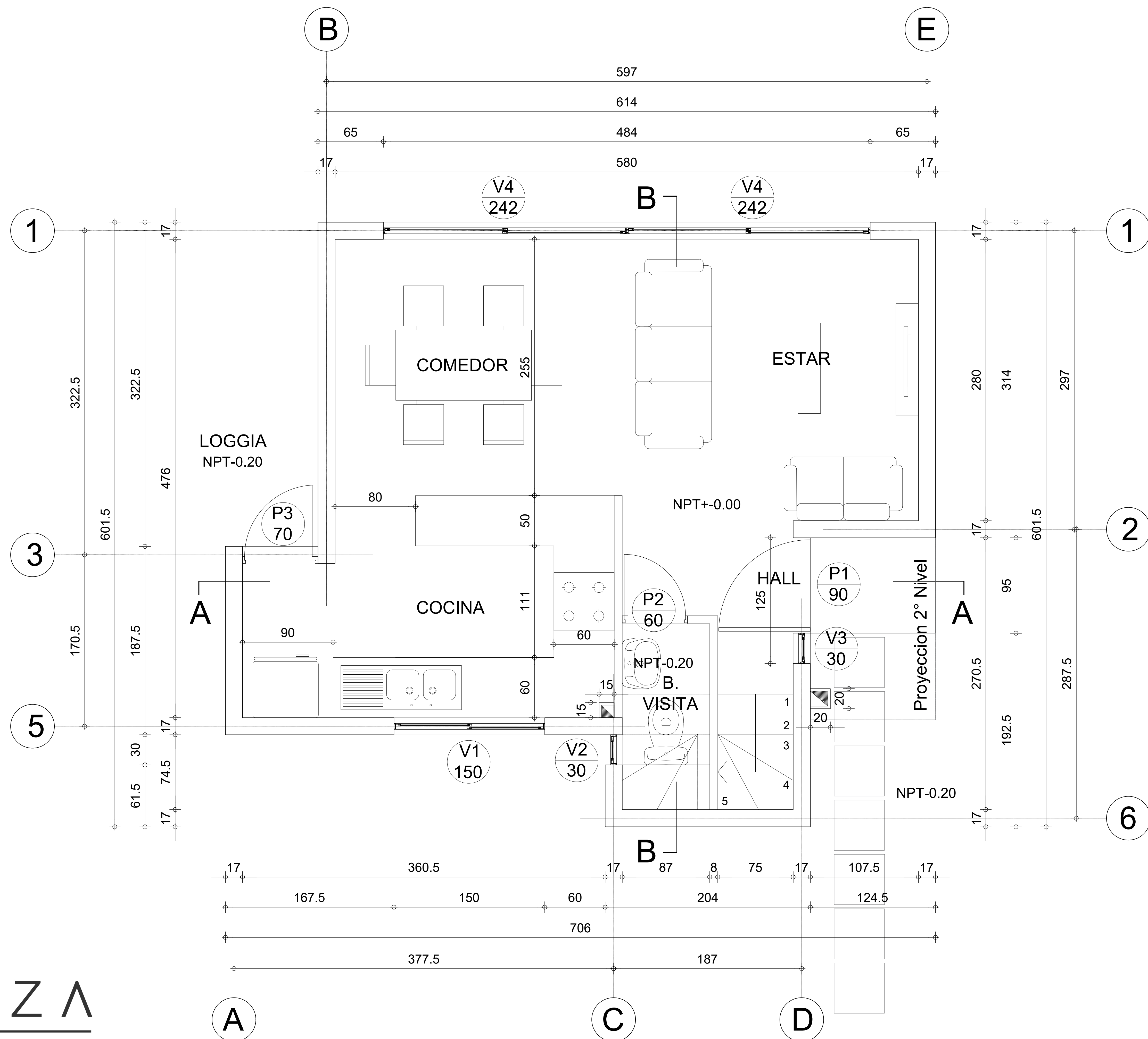
PLANTA PRIMER PISO
